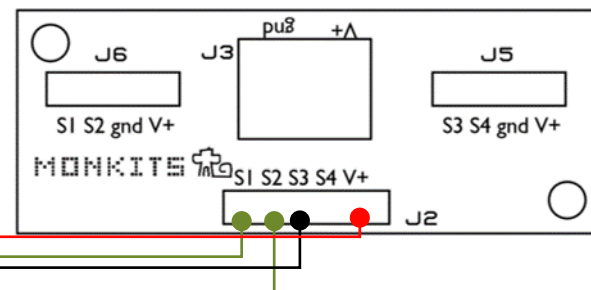
Puente H conexión a tarjeta joystick
